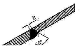
KAYNAK DETAYI ÇEK=1/1
